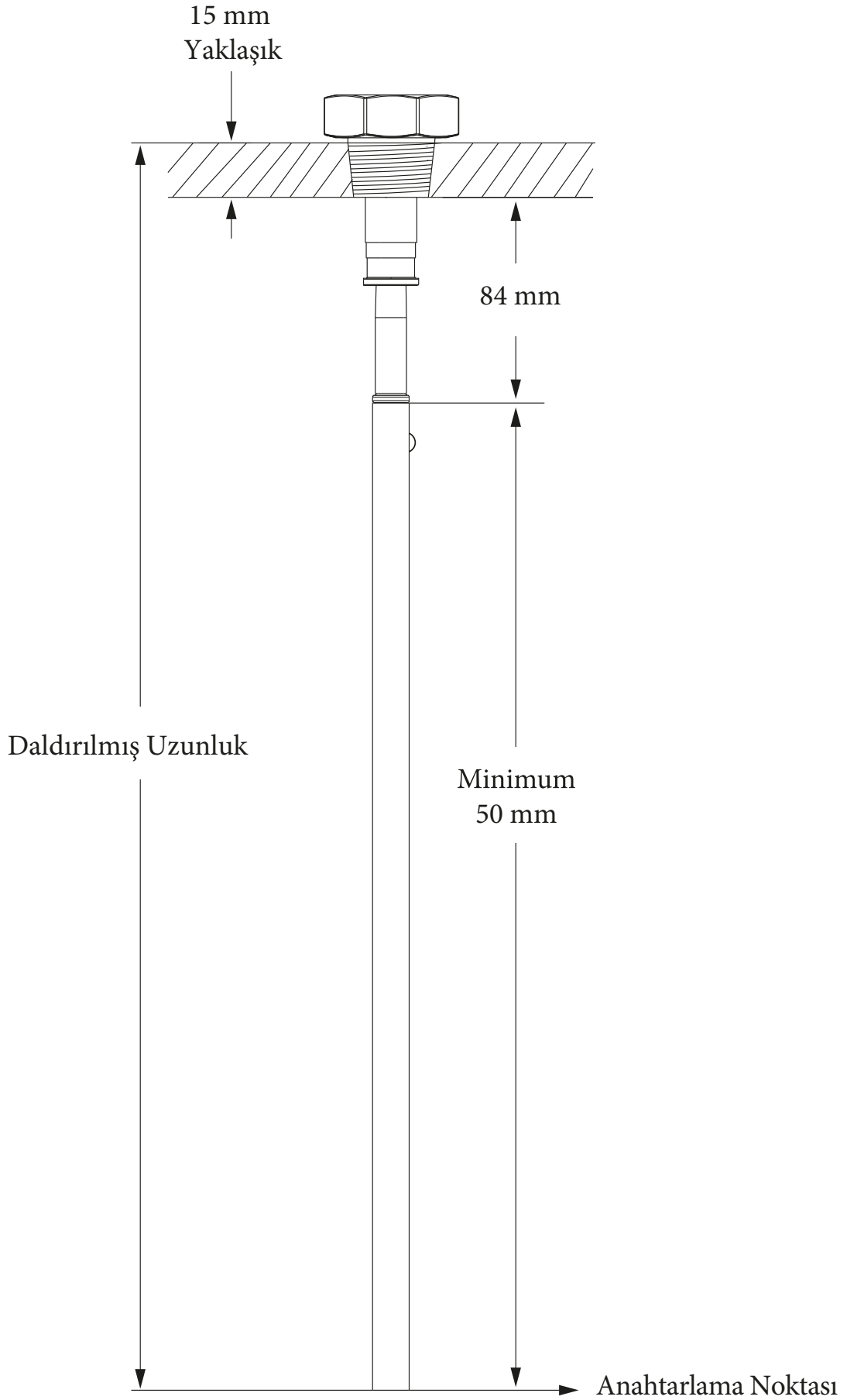
Şekil 6 : SMHD 1000 Elektrot uzunluk gösterimi
