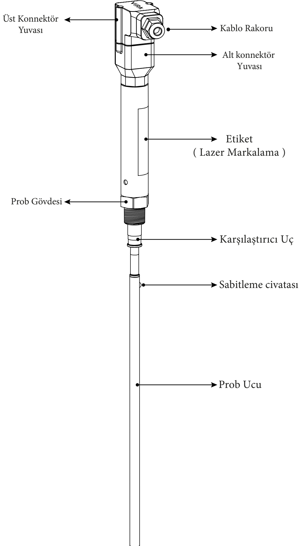
Şekil 2 : SMHD 1000 Malzeme Tanımı
