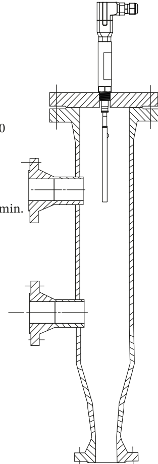
Şekil 5 : Kurulum örneği 3, koruma tüpü kazanın dışında olacak şekilde kullanım.
