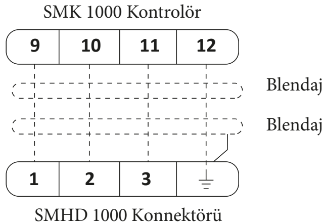
Şekil 8 : Bağlantı Şeması
